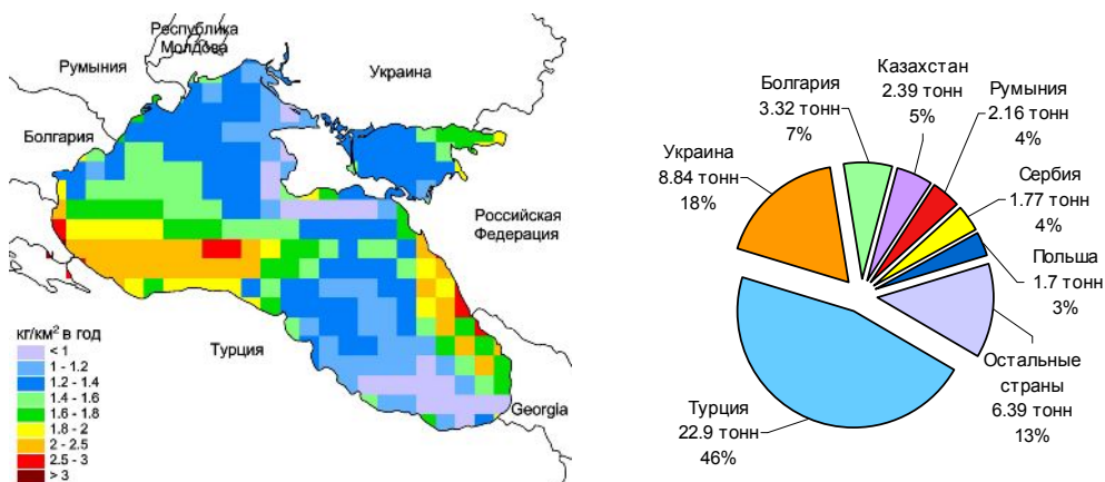
Рис. 4.17а. Пространственное распределение атмосферных выпадений ( \text{кг/км}^2 в год) и вклад стран Европы и Центральной Азии в атмосферное выпадение
