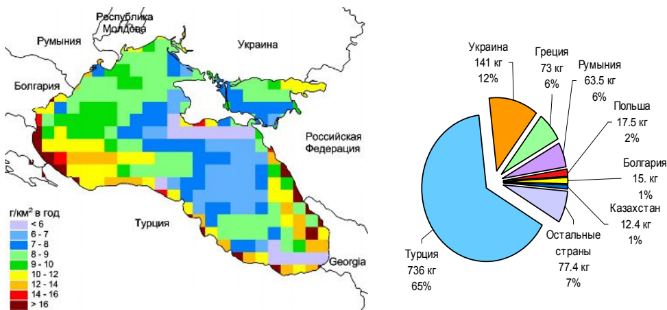
Рис. 4.17в. Пространственное распределение атмосферных выпадений (кг/км 2 в год) и вклад стран Европы и Центральной Азии в атмосферное выпадение ртути от антропогенных источников на акваторию Чёрного и Азовского морей в 2010 г.
