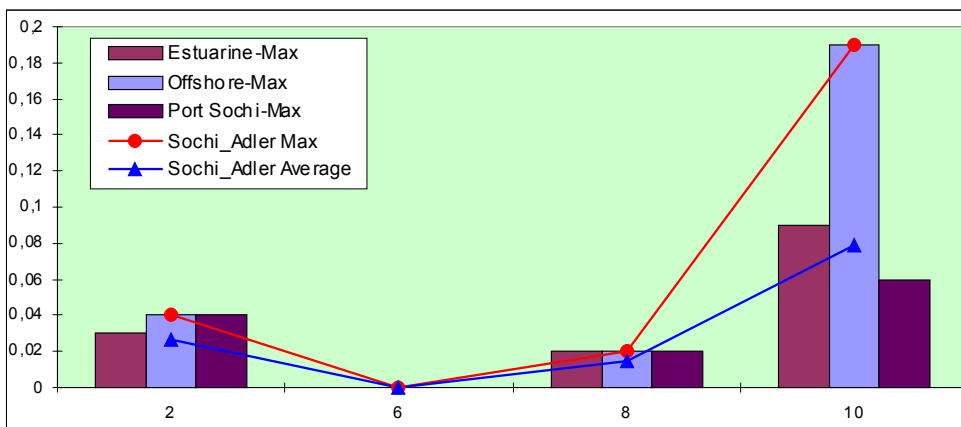
Рис. 4.16. Сезонные изменения максимальной и средней концентрации углеводородов (мг/л) в прибрежных водах района Адлер-Сочи в 2010 гг.
