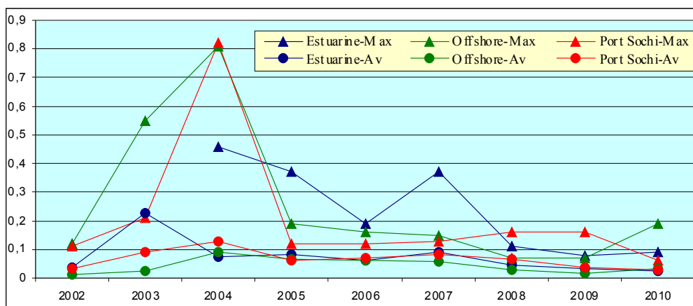
Рис. 4.15. Максимальная и средняя концентрация нефтяных углеводородов в прибрежных водах района Адлер-Сочи в 2002-2010 гг.
