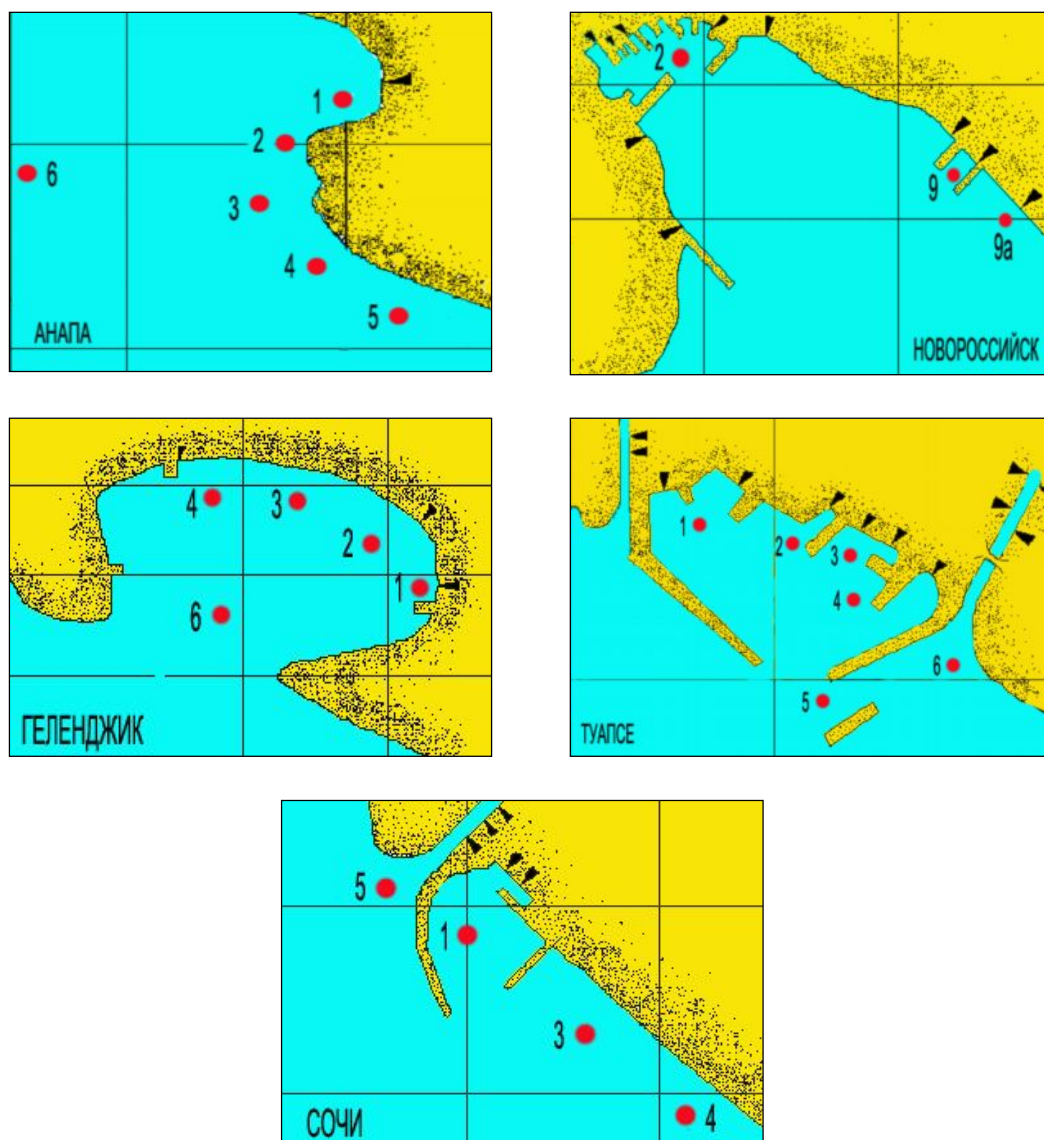
Рис. 4.1. Схема расположения станций отбора проб на акватории портов российской части Черного моря в 2006 г. (ГМБ Туапсе).
